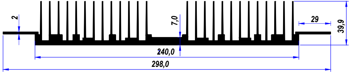
ADS - 298 Alm.Soğt.Prf. ÖLÇEK 1/2
