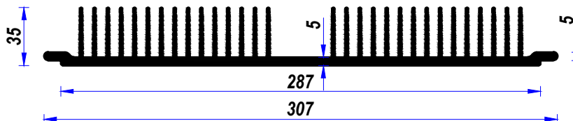
ADS - 307 Alm.Soğt.Prf. ÖLÇEK 1/3
