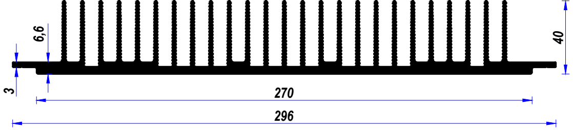
ADS-296 A Alm.Soğt.Prf. ÖLÇEK 1/2
