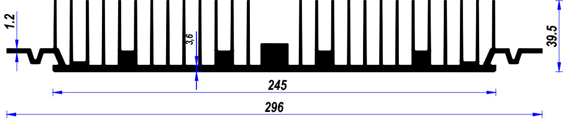
ADS - 296 Alm.Soğt.Prf. ÖLÇEK 1/2
